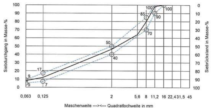
Sieblinienbereich für AC 11 D S
