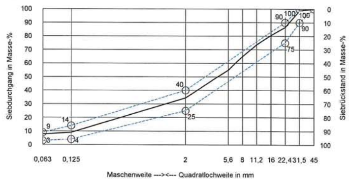
Sieblinienbereich für AC 32 T N
