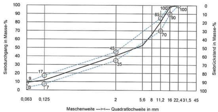
Sieblinienbereich für AC 16 D S
