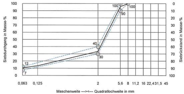
Sieblinienbereich für SMA 5 N
