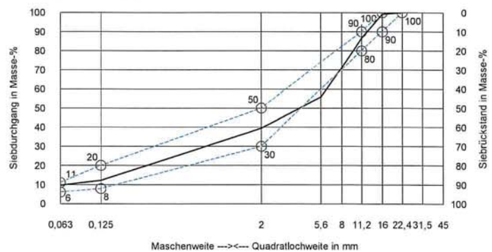
Sieblinienbereich für AC 16 TD
