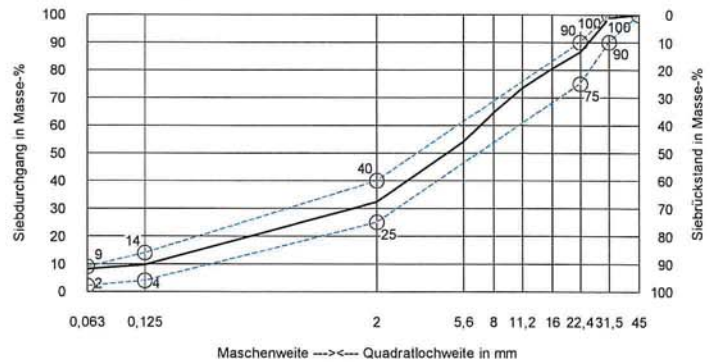
Sieblinienbereich für AC 32 T S
