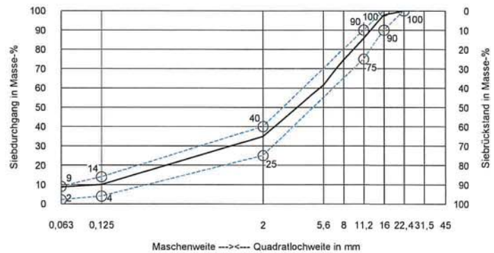
Sieblinienbereich für AC 16 T S
