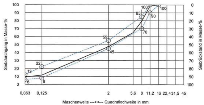
Sieblinienbereich für AC 11 D N
