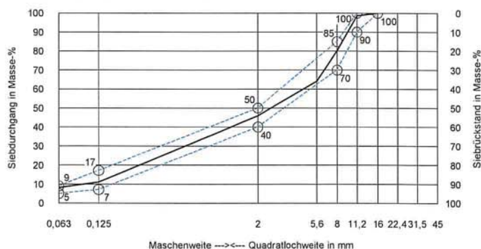
Sieblinienbereich für AC 11 D S
