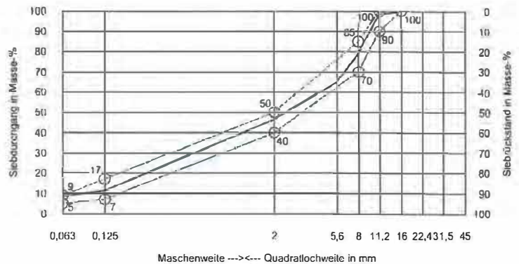
Sieblinienbereich für AC 11 D S
